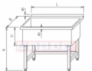
Typowe wymiary basenu (B-1000) x (L-500) x h
